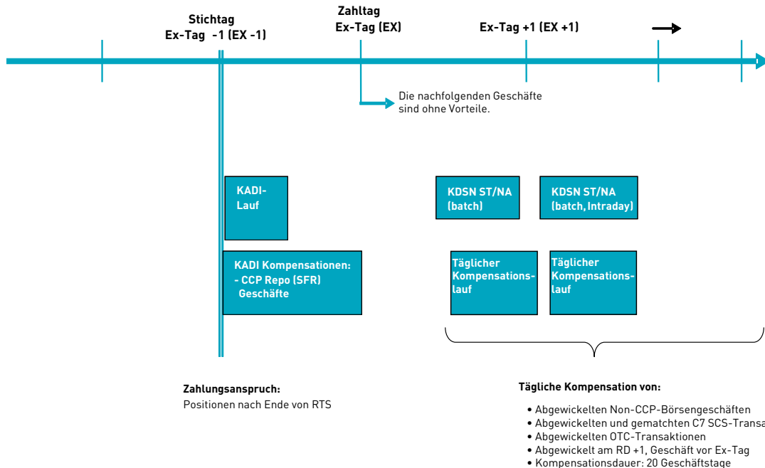
Abbildung 3.2 "Record Tag"-Verarbeitung von Terminart 120
