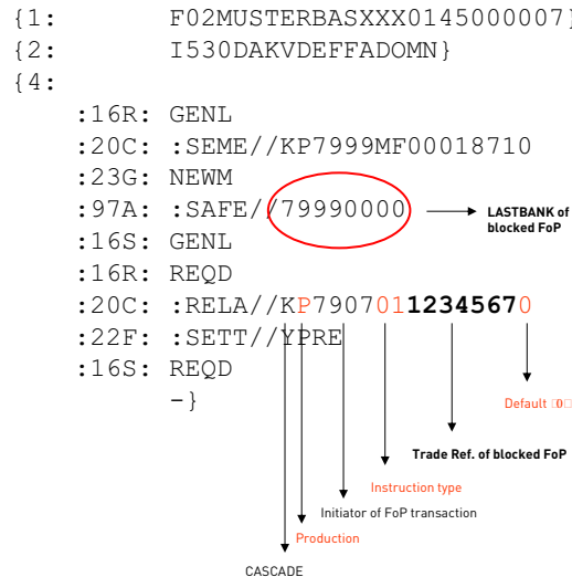
Abbildung 4.2 MT530 zur Freigabe von gesperrten FoP-Auträgen
