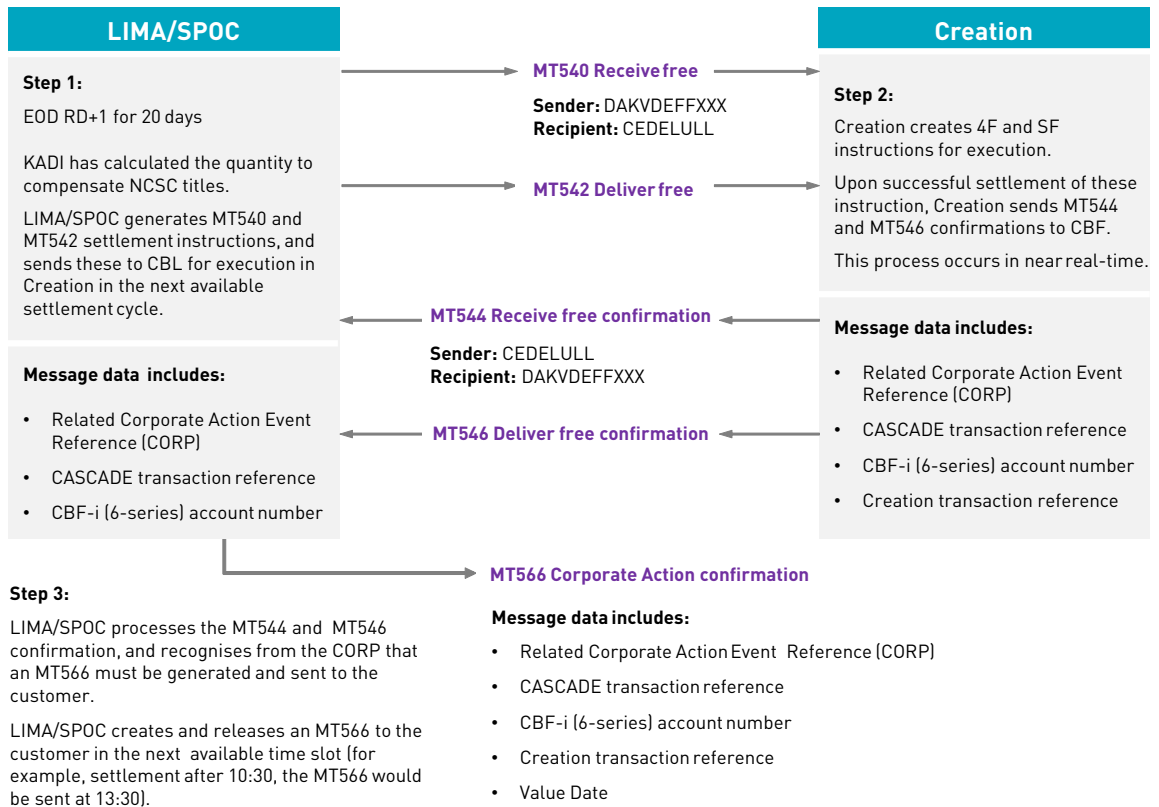
Abbildung 4.6 Prozess für Market Claims für Non-Income Events in AKV-Titeln (Creation)
