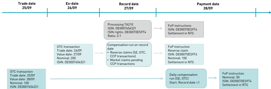
Abbildung 4.4 Market und Reverse Claim Verarbeitung von Terminart 210 (Ausgabe Bezugsrecht mit „Record Tag“-Verarbeitung)
